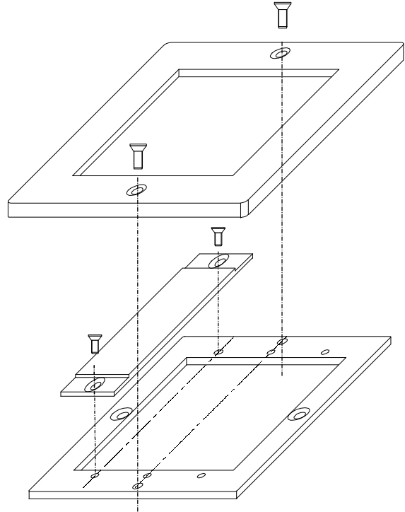
Abdeckrahmen (6 Slotbreiten) (863 9201)
